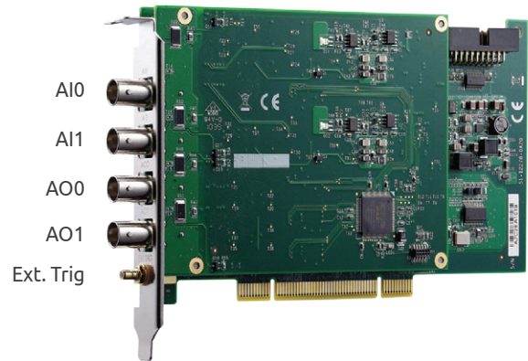
PCI-9527L
